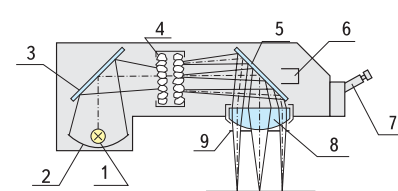
Рис. 8. Блок экспонирования
