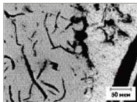
Рис. 9. Чешуйки графита в сером литейном чугуне
