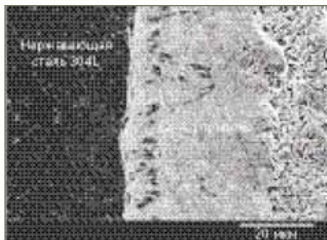
Рис. 2. Изображение точечной коррозии, полученное сканирующим электронным микроскопом
