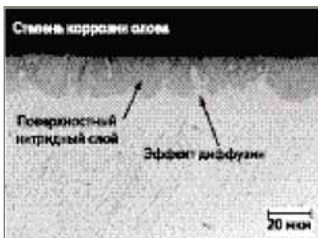
Рис. 7. 50-кратное изображение образца из нержавеющей стали AISI 316 с покрытием Melonite®, полученное с помощью оптического микроскопа
