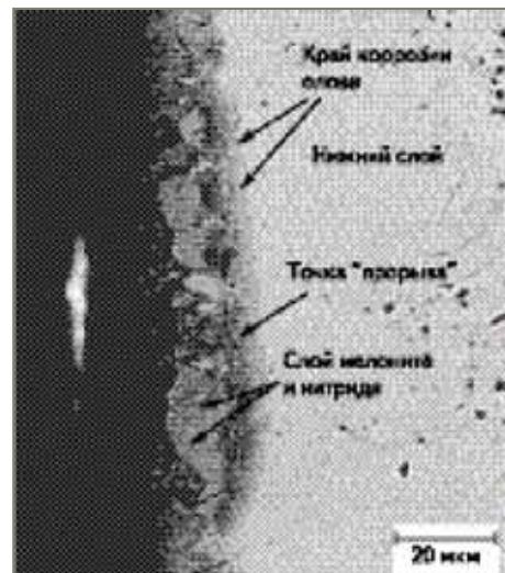
Рис. 8. Протравливание при температуре 350 °C
