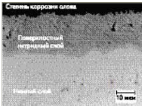
Рис. 6. 100-кратное изображение образца из нержавеющей стали AISI 304 с покрытием Melonite®, полученное с помощью оптического микроскопа
