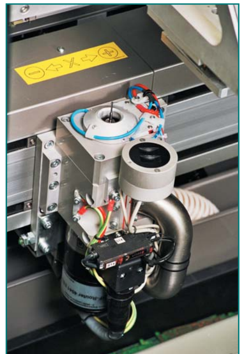
Рис. 15. Фреза высокоскоростного роутера J501-41
