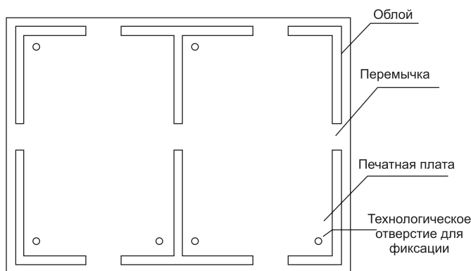
Рис. 5. Пример построения групповой заготовки
