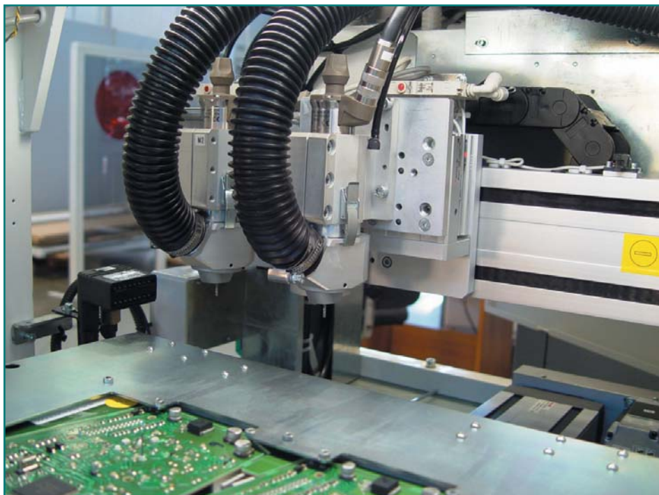
Рис. 3. Разделение групповых заготовок фрезой вертикального типа
