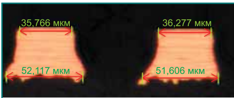
Рис. 7. Рисунок, полученный на горизонтальной травильной установке
