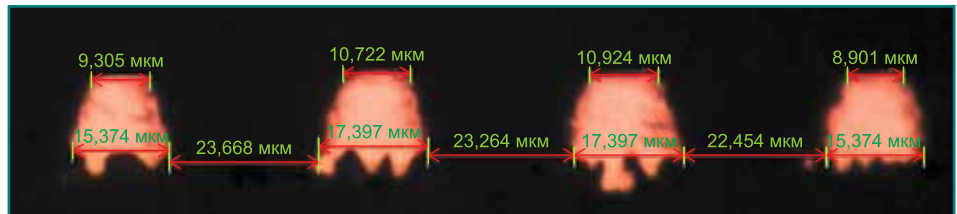
Рис. 8. Рисунок, полученный на вертикальной травильной установке
