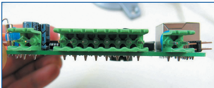
Рис. 6. Использование клемм WJ2EDGR на печатной плате
