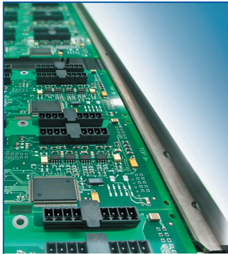
Рис. 14. Клеммы из LCP на плате с пластиной для захвата манипулятором
